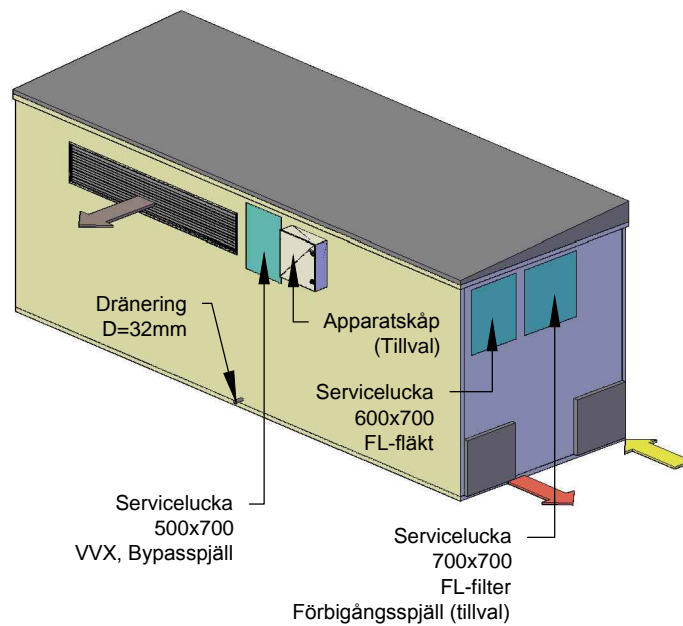
(1:75) 3D Vy framifrån höger
