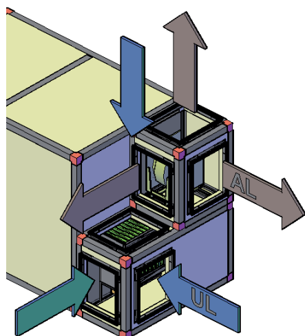
Anslutningsmöjligheter Uteluft/Avluft
