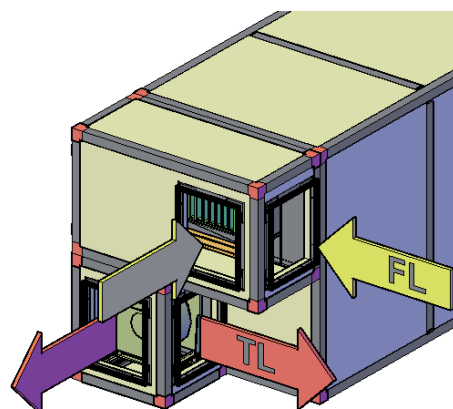
Anslutningsmöjligheter Tilluft/Frånluft
